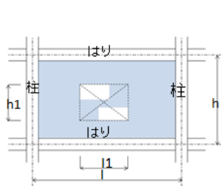
高さ h_1 、長さ l_1 の開口とみなす
