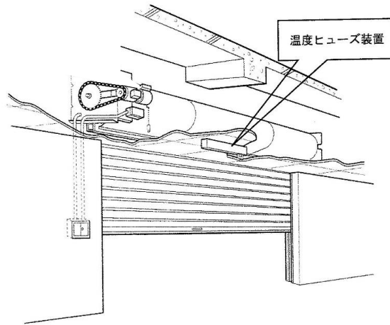
温度ヒューズ式防火シャッターの例
