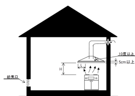
(d) 排気フードⅡ型
