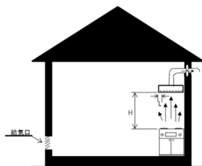
(c) 排気フードⅠ型
