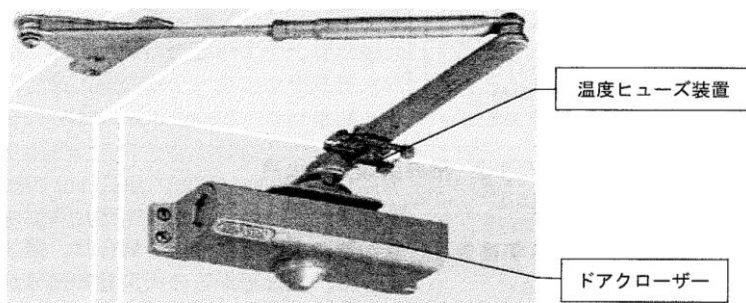
温度ヒューズ付ドアクローザー例
